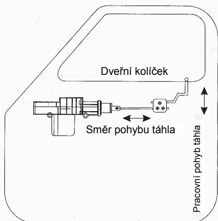
Horizontální instalace
