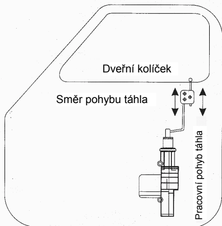
Vertikální instalace
